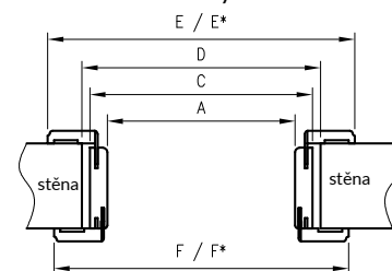
Vodorovný řez
