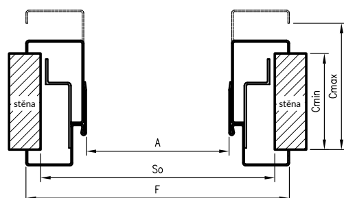
S0 - šířka montážního otvoru
