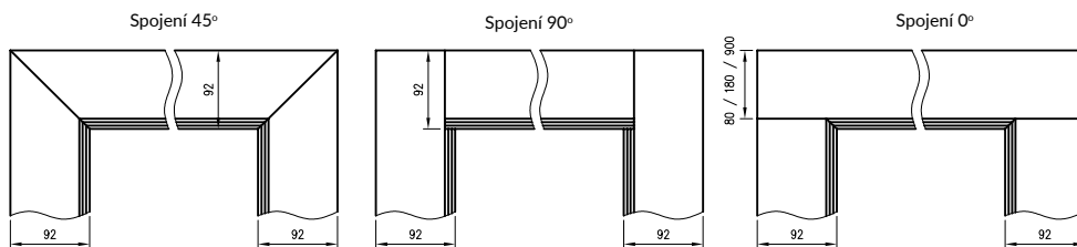
Průřez ORB
