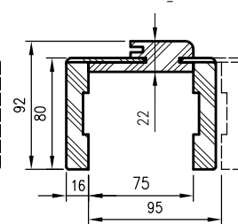
Průřez ORB_075
