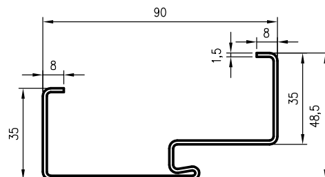
Profil zárubně
