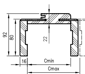
Průřez ORB
