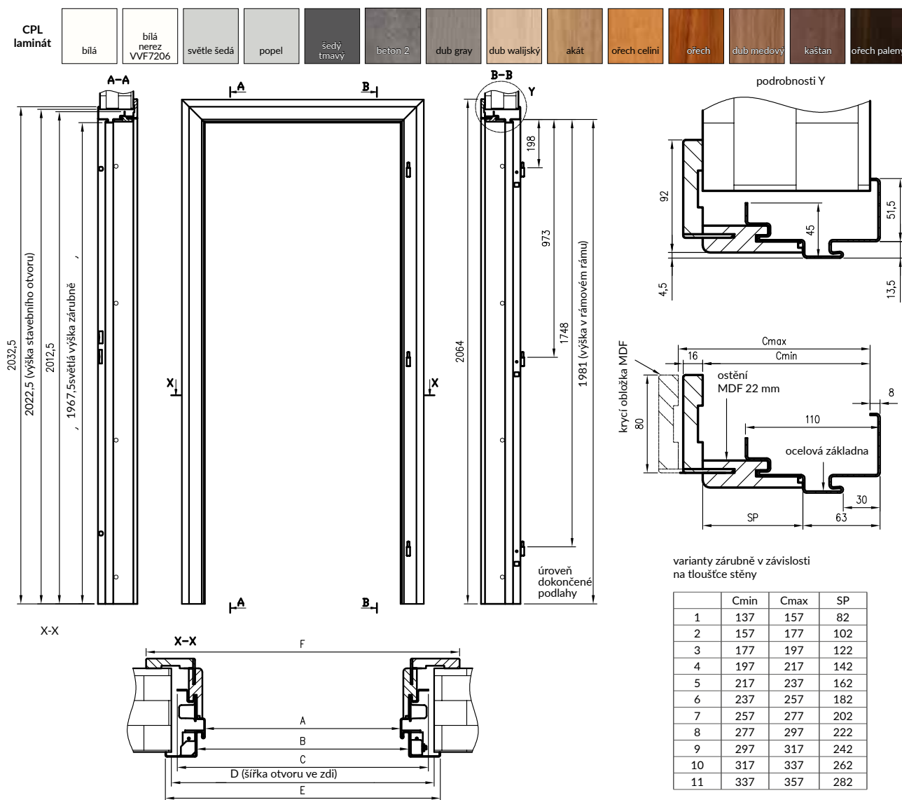
příklady barevných kombinací ocelové hybridní zárubně
