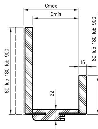
Průřez ORB_075
