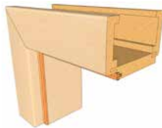
Řez obložkovou zárubní (OKZ) přes původní kovové zárubně síla zdi od 50 mm, límce 80 mm
