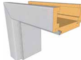
Řez obložkovou zárubní Kovolaminát síla zdi od 100 mm, límce 60 mm
