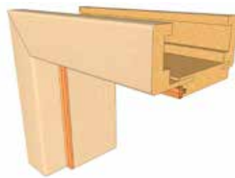
Řez obložkovou zárubní pro otočné bezfalcové dveře síla zdi od 100 mm, límce 60 mm
