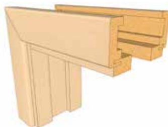
Řez obložkovou zárubní pro stavební pouzdra síla zdi od 100 mm, límce 60 mm
